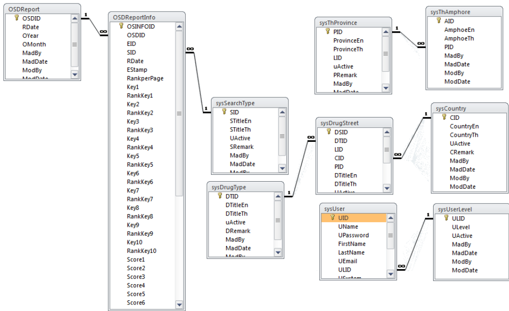
ภาพ 1 แสดงลักษณะโครงสร้างและความสัมพันธ์ระหว่างตารางข้อมูล
